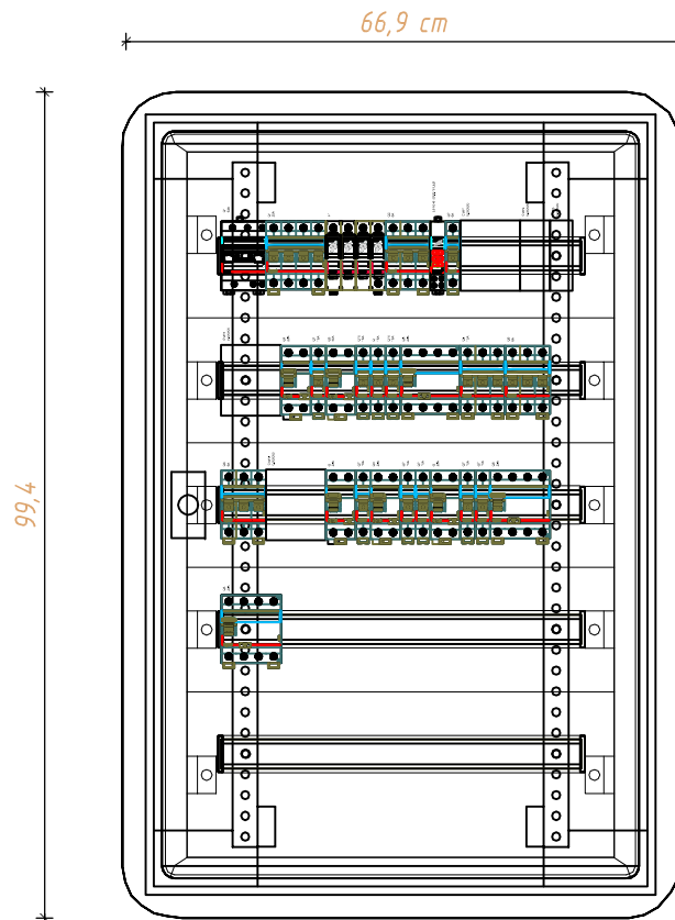
Rozdzielnica wtynkowa, izolacyjna, wyposażona, np. XL 3 160, 5x24 mod., drzwiczki płaskie, metalowe, montaż na wysokości ok. 105 cm od posadzki.
